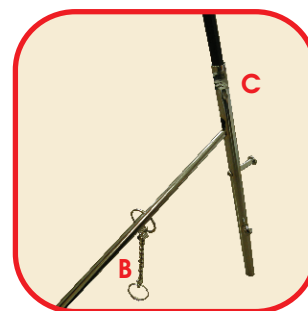
2. Sujunkite atraminę kojelę su apatiniais strypais.
