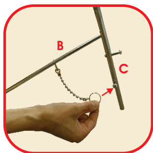
3. Užkabinkite grandinėles už strypų.
